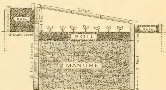
FIG. 27. A simple hotbed. (Erwin.)
